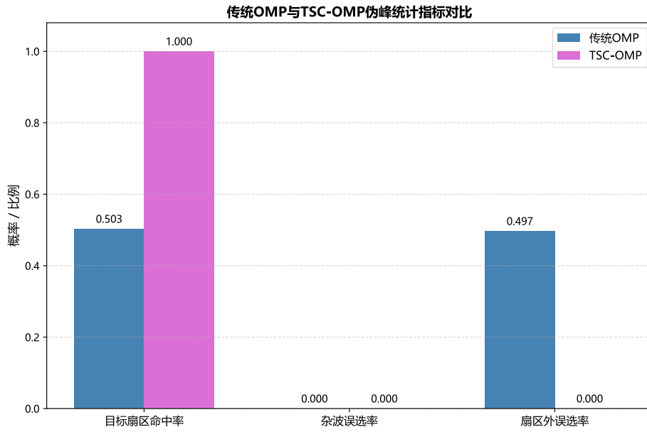
图 4-3 传统 OMP 与 TSC-OMP 伪峰统计指标对比
