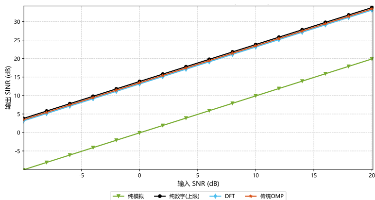
图 3-3 非均匀线阵下各算法的 SINR 表现
