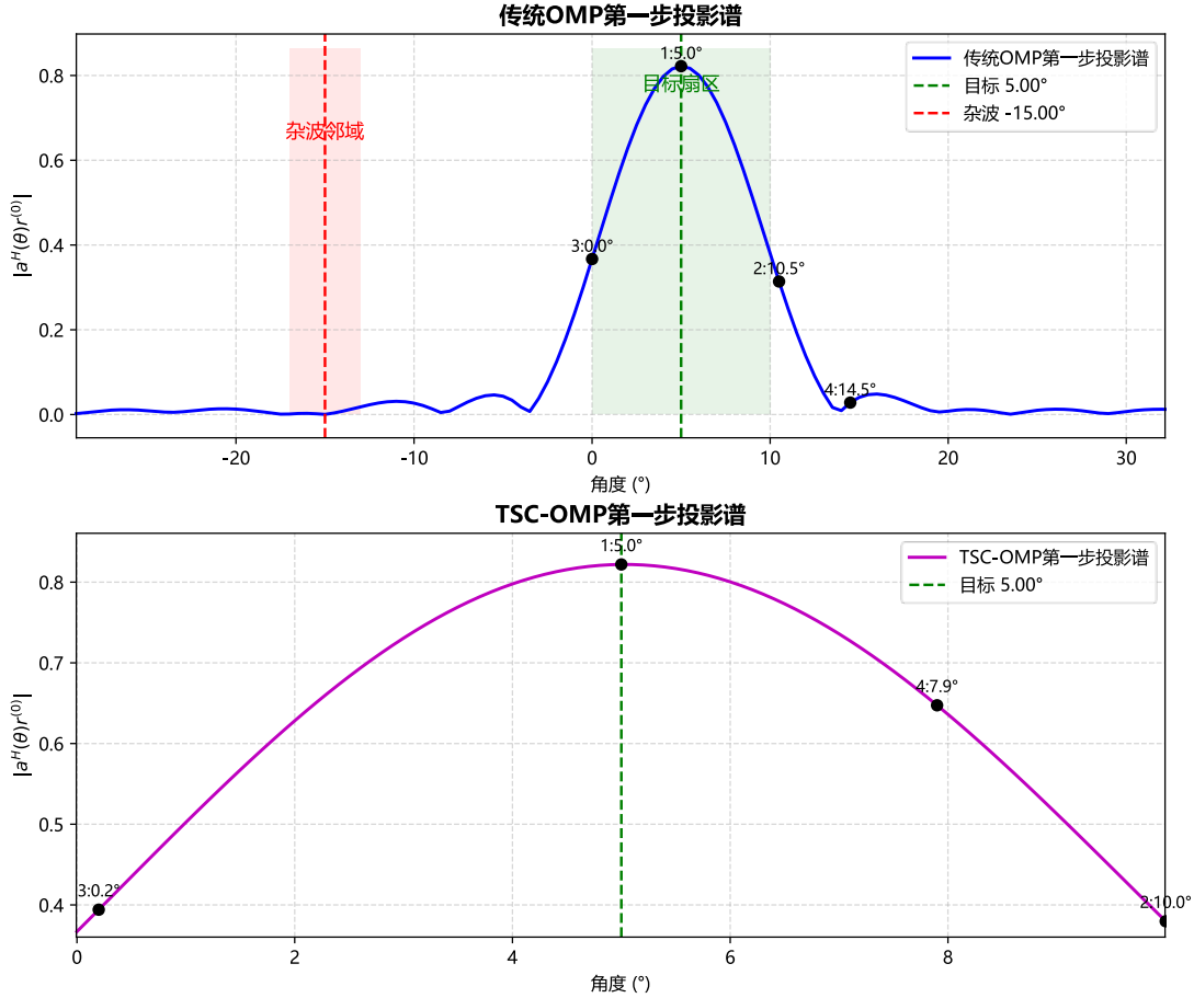
图 4-1 传统 OMP 与 TSC-OMP 第一步投影谱对比
